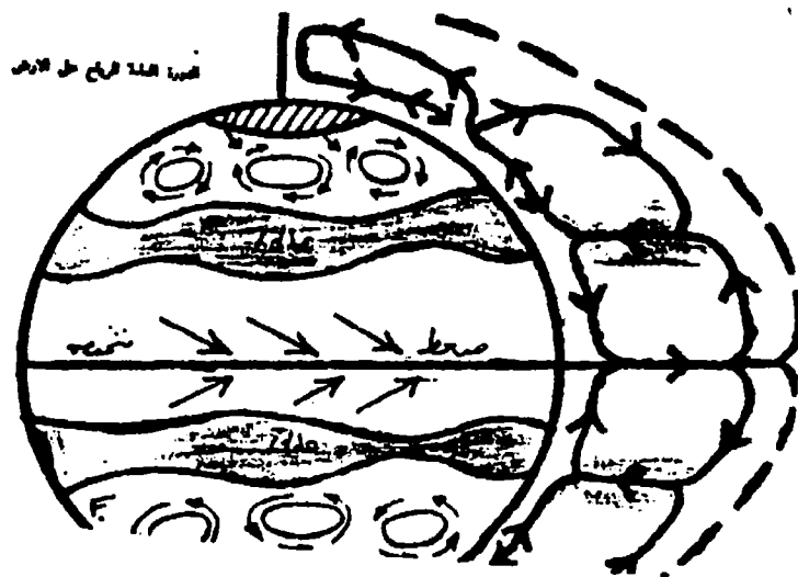
الدورة العامة للرياح على الأرض
